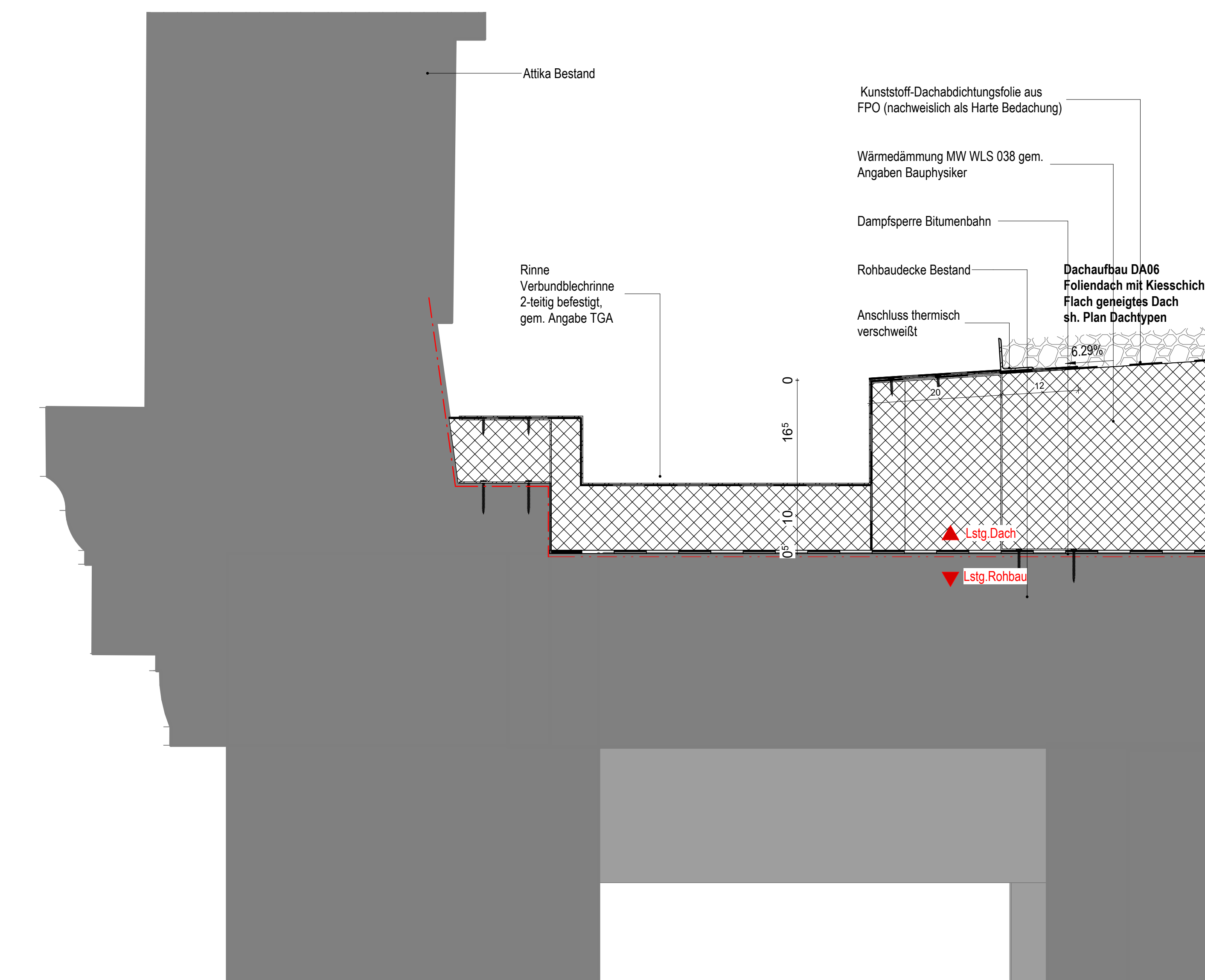
Bestandsgebäude Magazinswest Rinne 1 : 5
