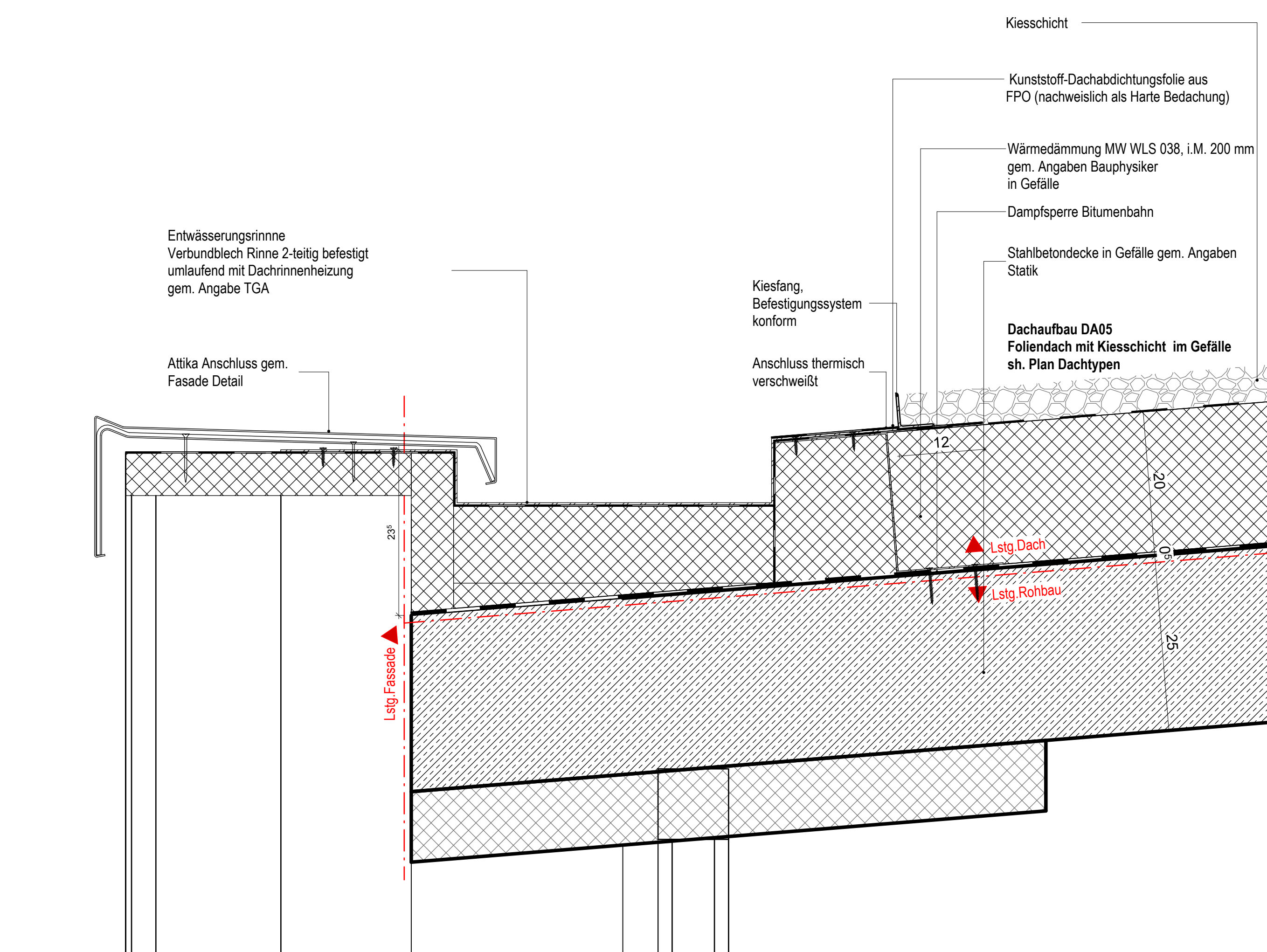
KH_Dach Rinne 1 : 5
